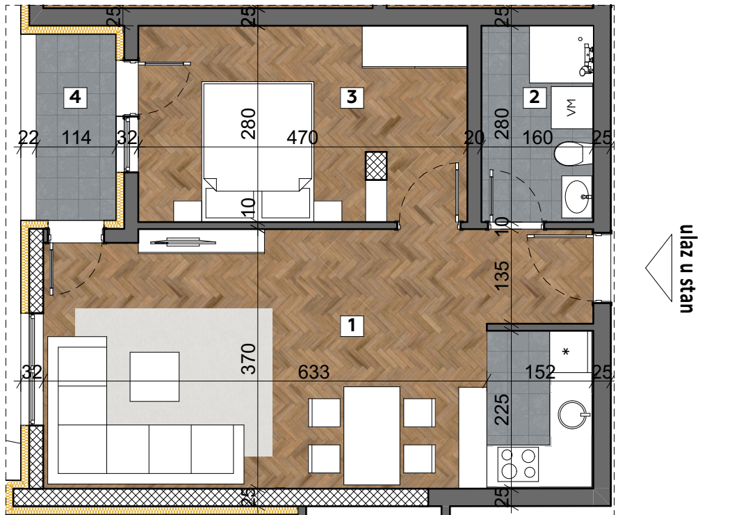
osnova stana
